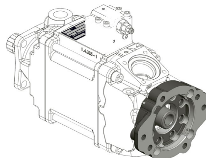
11465010162 Applicazione PPV60 tandem / Pompa SAE B Z13 (coppia trasmissibile 210Nm) PPV tandem 60 size / SAE B Z13 pump adaptor (max. allowed torque 210Nm)
