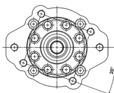
11465010162 Applicazione PPV60 tandem / Pompa SAE B Z13 (coppia trasmissibile 210Nm) PPV tandem 60 size / SAE B Z13 pump adaptor (max. allowed torque 210Nm)
