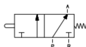
Schema di funzionamento Functional diagram
