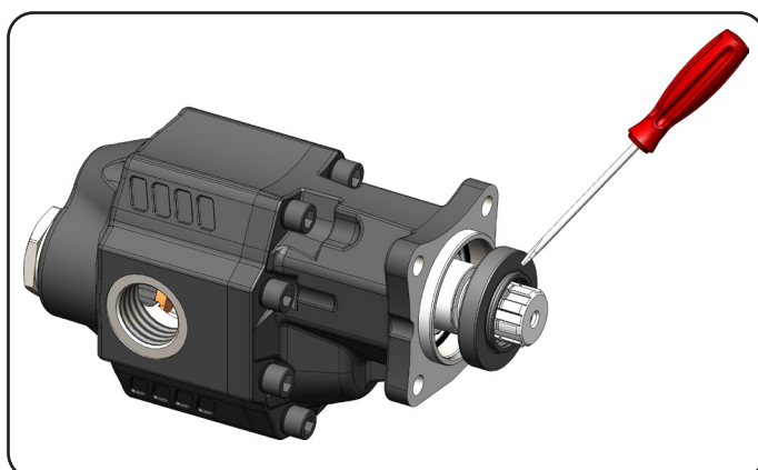
Fig. 2 Togliere il paraolio Remove the oil seal
