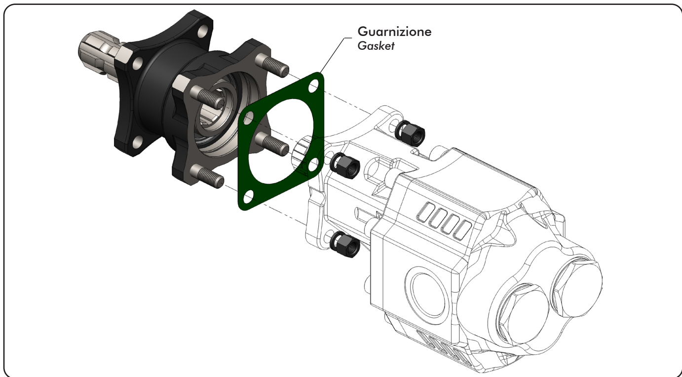
Fig. 3 Montare il supporto alla pompa interponendo la guarnizione a corredo. Mount the bracket on the pump and interject the gasket provided.
