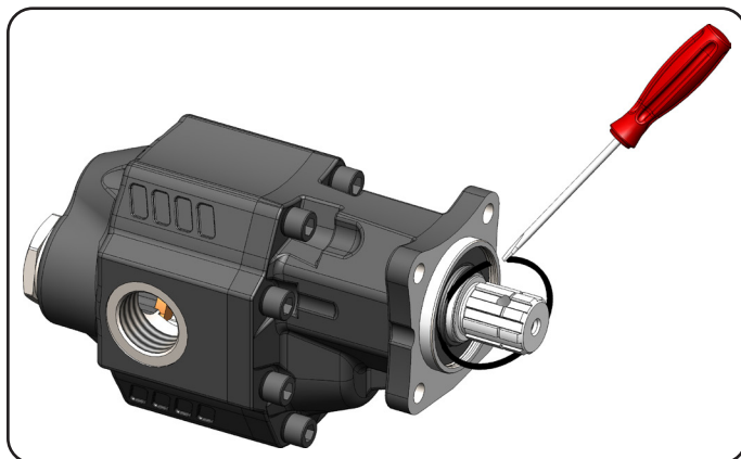
Fig. 1 Togliere il seeger Remove the seeger
